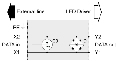
G3 : Descargador tripolar D : Diodo limitador
